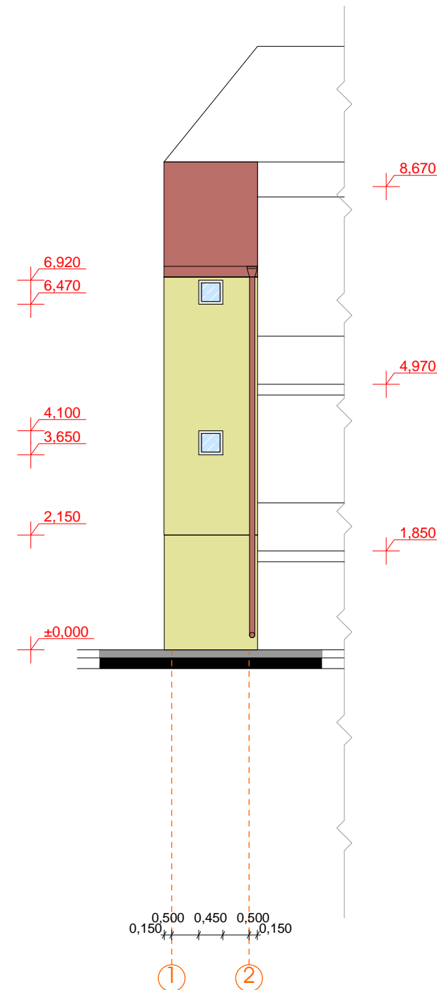
განშლა 1-2 ღერძებში
