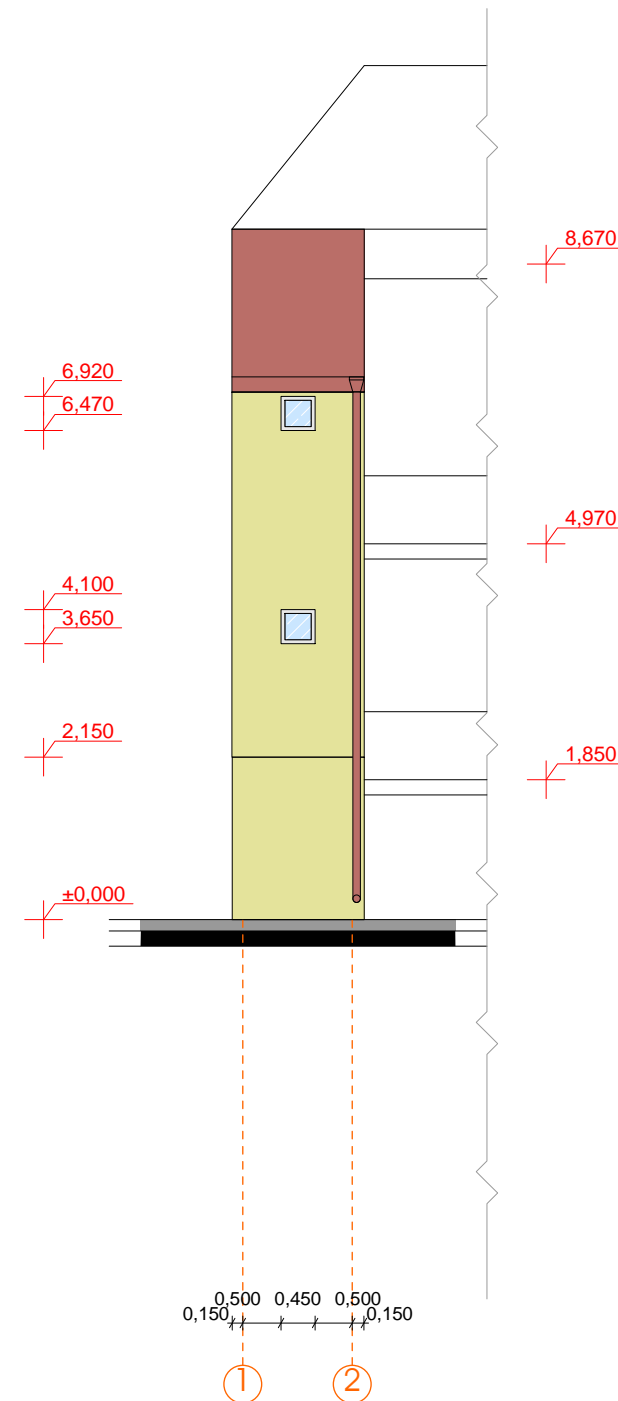
ბანსა 1-2 ღერძებში
